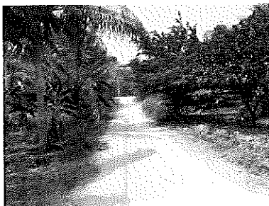
โครงการ ก่อสร้างถนนคอนกรีตเสริมเหล็ก สายชอยโกรกกรือ ช่วงที่ ๓ ม.๕
