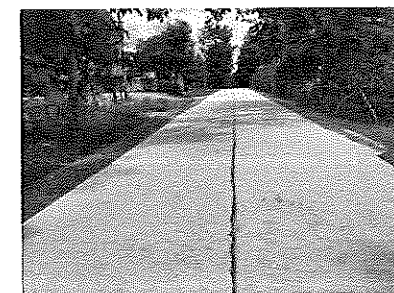
โครงการ ก่อสร้างถนนคอนกรีตเสริมเหล็ก สายชอย ๑๖ ม.๗
