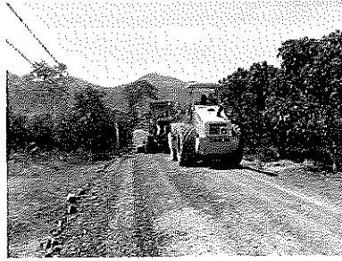
โครงการก่อสร้างถนนหินคลุก สายซอยมรกต ม.๔
